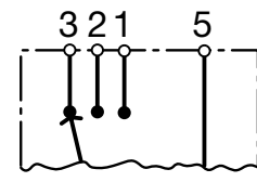
Spannungswähler 3-stellig 2-polig
